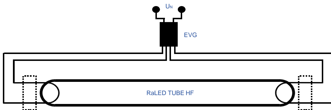
Schaltbild einer umgerüsteten EVG-Leuchte
